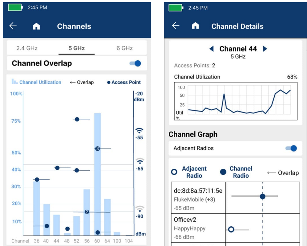
Gauche : Utilisation de chaque canal sur la bande passante de 5 GHz, avec affichage des AP et du chevauchement pour chacun d'entre eux. Droite : Les détails d'un canal individuel montrent l'utilisation dans le temps et les détails des radios qui chevauchent ce canal.
