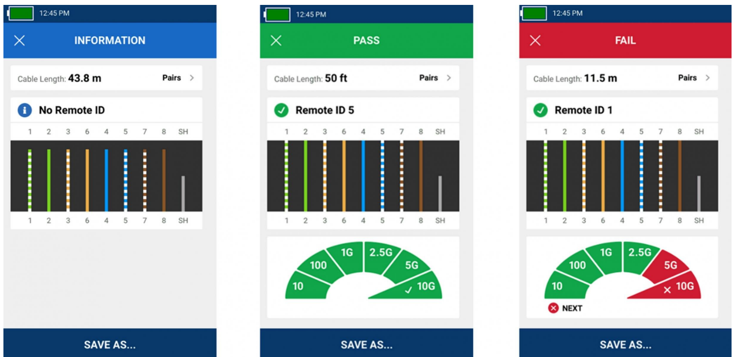
Gauche : Le test de câble sans connexion à distance indique la longueur et l'appariement de chaque fil. Centre : Le test de câble avec connexion à distance indique le numéro d'identifiant distant 5, la longueur et l'appariement de chaque fil et les performances du câble jusqu'à 10 Gb/s. Droite : le test de câble avec l'unité distante indique l'identifiant distant numéro 1, la longueur et l'appariement de chaque fil et les performances de câble jusqu'à 2,5 Gb/s, mais le test a échoué en raison d'une limite de performance de 10 Gb/s définie par l'utilisateur.
