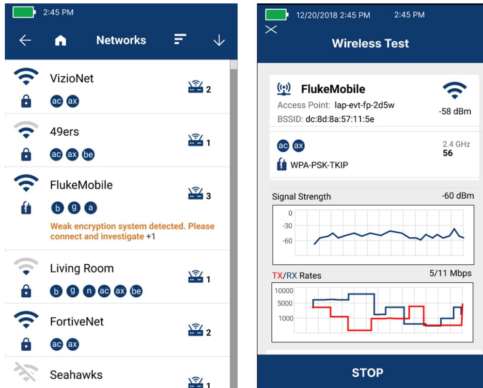
Gauche : Détails du réseau indiquant l'AP le plus proche, la puissance du signal, les radios, le résumé de la bande/du canal, la technologie et le cryptage. Droite : le test du point d'accès montre la force du signal et les débits de données au fil du temps.
